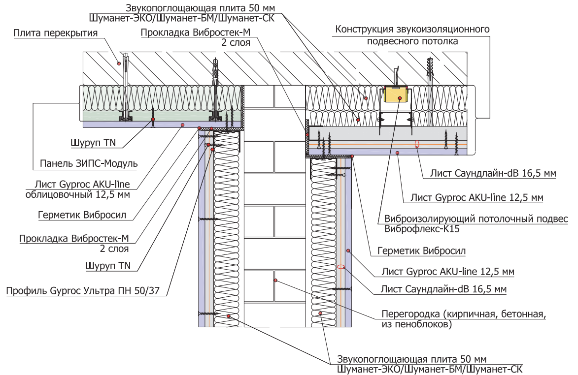
3.1.3 Угловое примыкание облицовки стены на независимом каркасе 50 мм к панелям ЗИПС на стене и дверному проему
